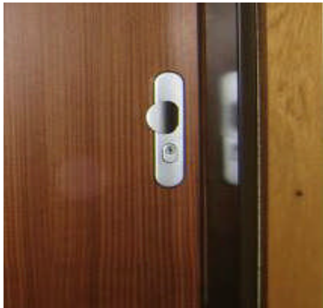
richtig: Sicherheitsschloss / bündige Blende und Blende ist nicht abschraubbar
